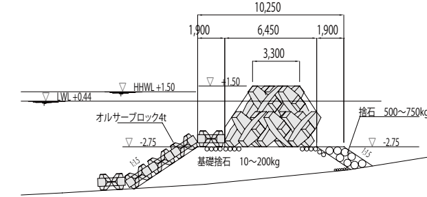
◇ 離岸堤被覆工 (2) : OR4t-I 型 (京都府宮津市 養老漁港海岸)
