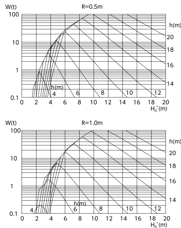
オルサーブロックの所要質量 (土研式)
