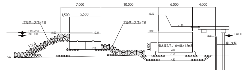
◇ 海水導入潜堤被覆工 : OR2t-I 型 (富山県富山市 四方漁港)
