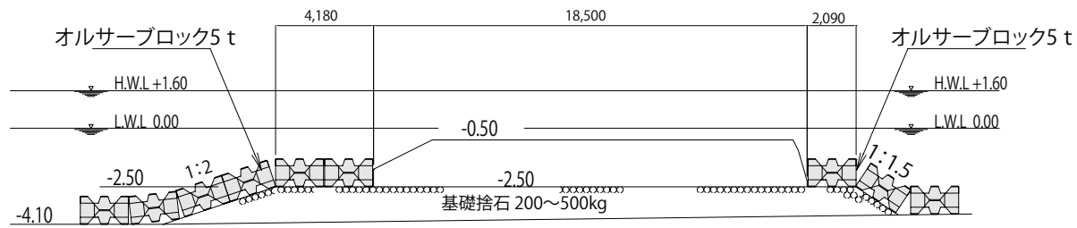
◇ 人工リーフ事例 (4) : OR-I 型5t溝型 (神奈川県葉山町 真名瀬漁港海岸)
