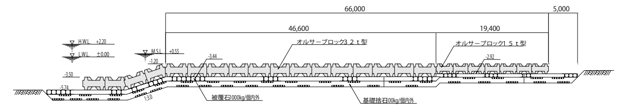
◇ 人工リーフ事例 (1)：OR-I型32t、15t (大分県 間越漁港海岸)
