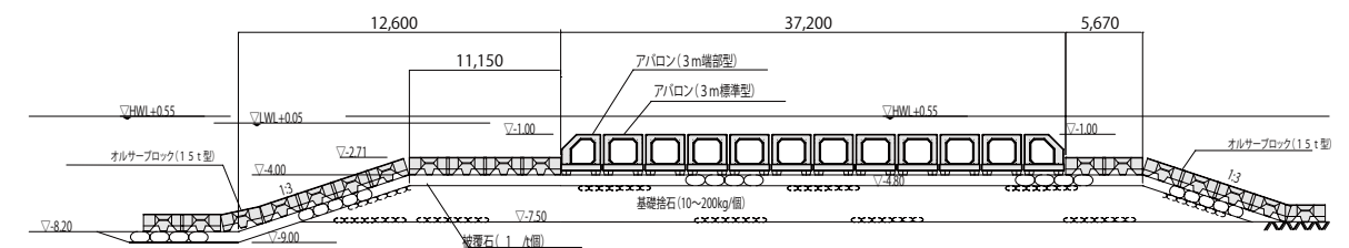
◇ 人工リーフ事例 (2)：OR-II型15t (兵庫県 香住漁港海岸)
