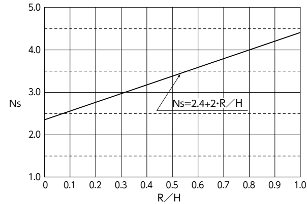
オルサーブロックの安定係数: Ns (人工リーフ)
