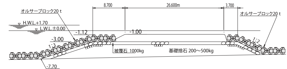
◇ 人工リーフ事例 (3)：OR-I型20t (東京都三宅島 三池港海岸)
