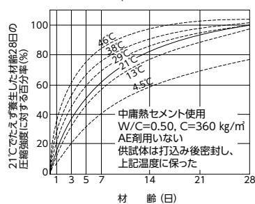
図2.2-6 養生温度と圧縮強度との関係 9)
