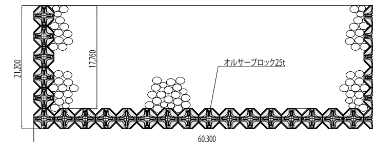
◇ 漁場整備囲礁工 : OR25t-I 型溝型 (山口県 豊岡沿岸地区漁場整備 : 4地区)
